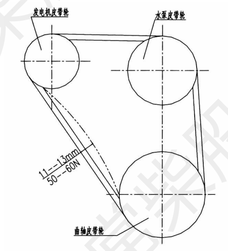
风扇皮带轮张紧度的调整示意图
