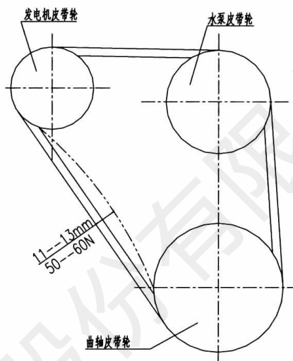
风扇皮带轮张紧度的调整示意图
